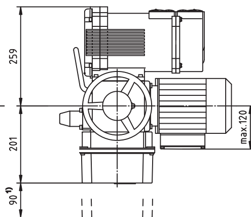
S řídící jednotkou SMARTCON
