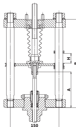
Připojení dle ISO 5210 Tvar A, F10, Tr36x6-LH NPS 1" - 3"
