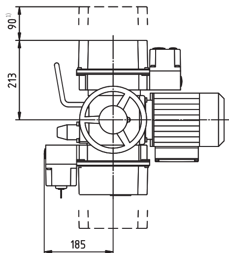
S regulátorem polohy ACTUMATIC R
