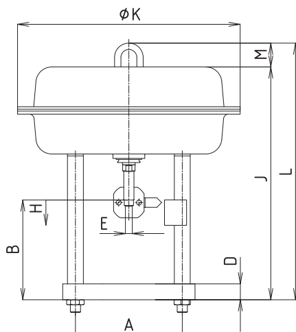
Standardní pohon
